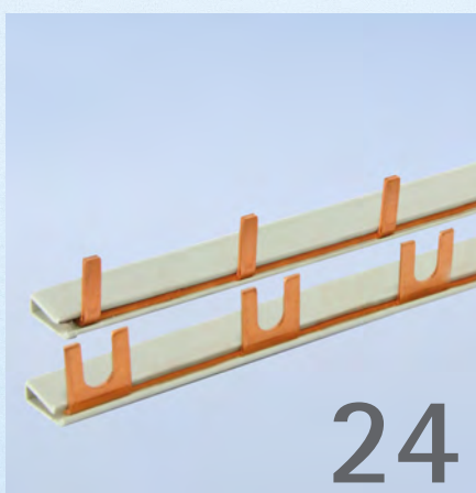
Phasenschiene für Hilfsschalter H1+H2 Busbars for Auxiliary switch H1+H2 Peignes unipolaires pour Interrupteur auxiliaire H1+H2
