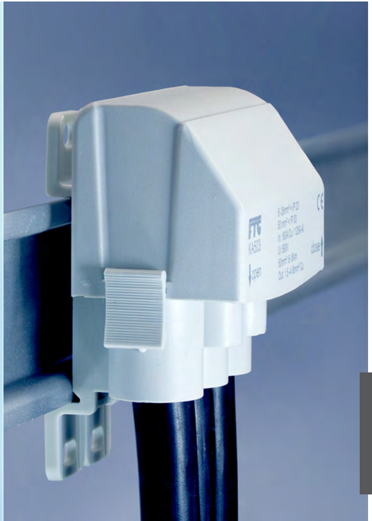
KA503 mit Halter KAH befestigt auf DIN-Tragschiene | KA503 with holder KAH mounted on DIN Rail | KA503 avec support KAH monté sur rail DIN
