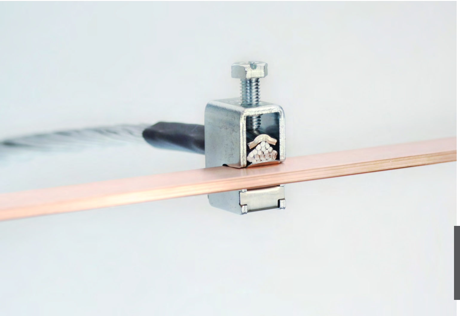
BKNA in Anwendung auf Kupfersammelschiene | BKNA in application on copper bar | BKNA en application avec rail de cuivre
