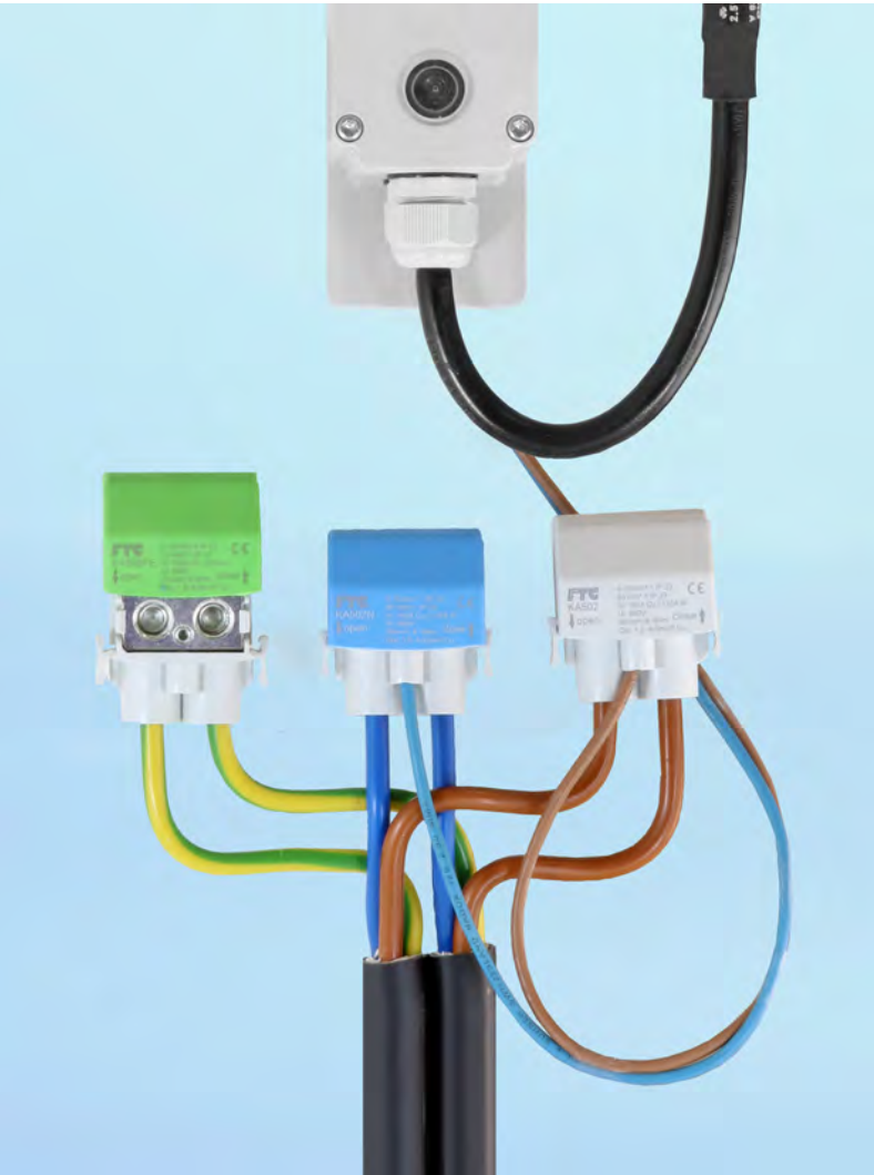
LPDB in Anwendung bei Straßenleuchten | LPDB in application for street lights | LPDB installé dans un lampadaire
