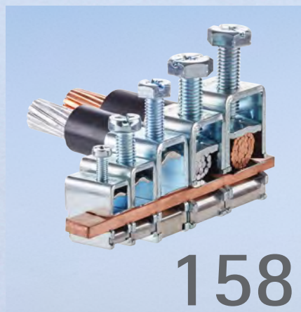
Stahlklemmen Steel terminals Bornes en acier
